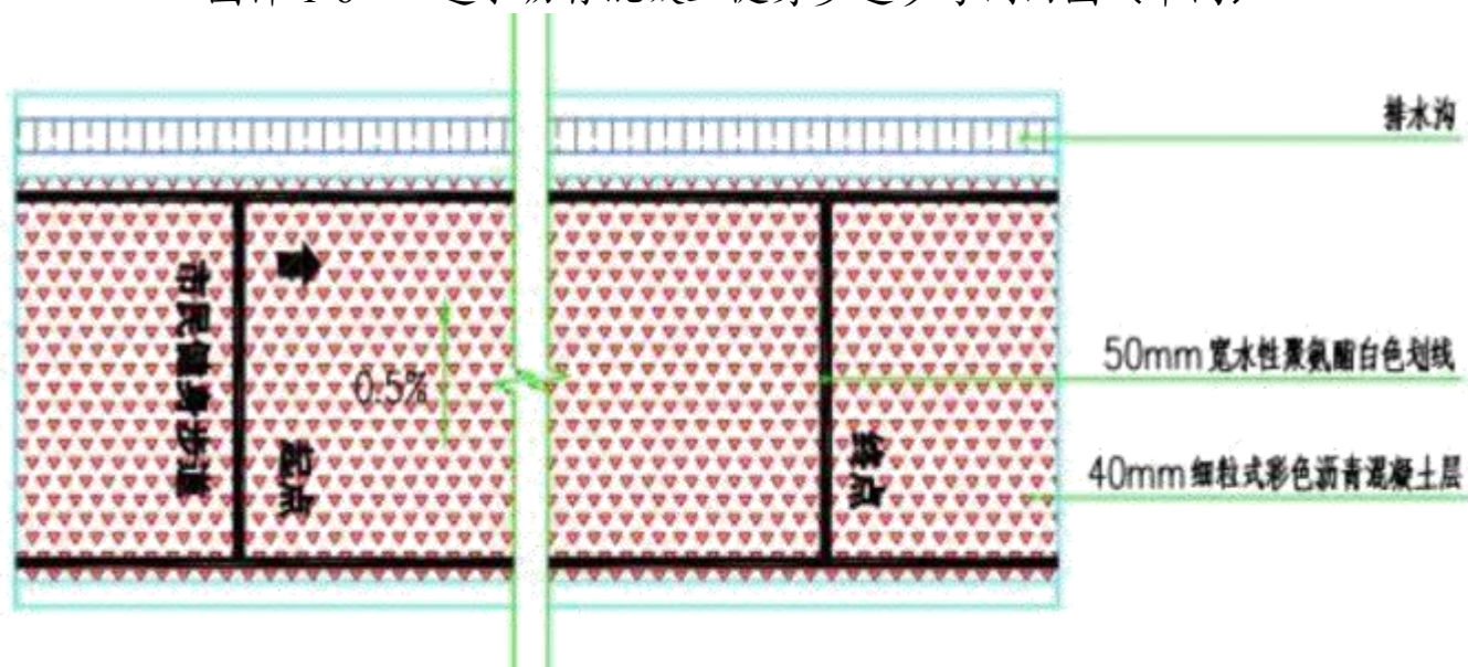
图件 1-6 透水沥青混凝土健身步道参考剖面图 (单向)
