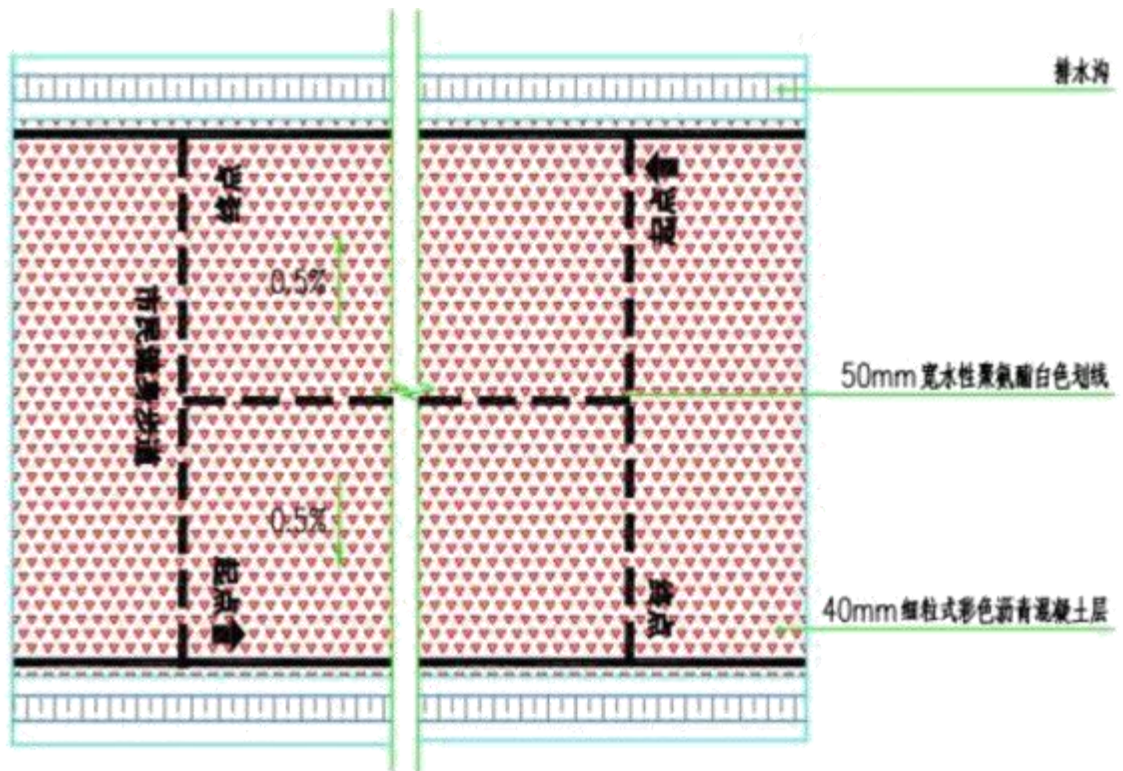
图件 1-13 彩色沥青混凝土健身步道参考平面图 (双向标准段)
