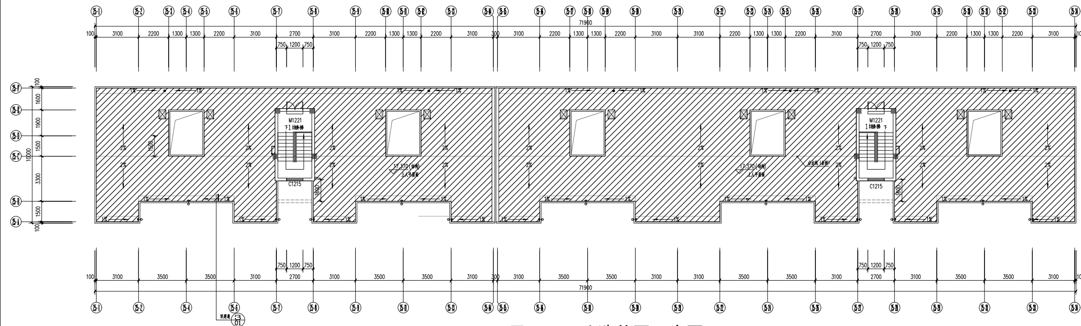
24#、25#屋顶平面改造范围示意图
