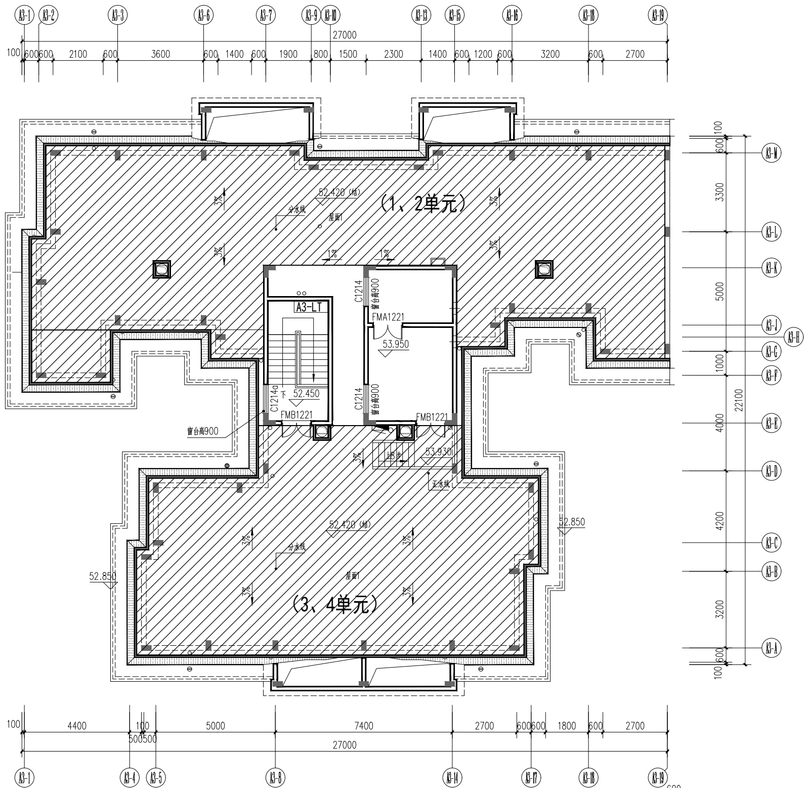
9#、10#、12#、13#标准单元屋顶平面改造范围示意图
