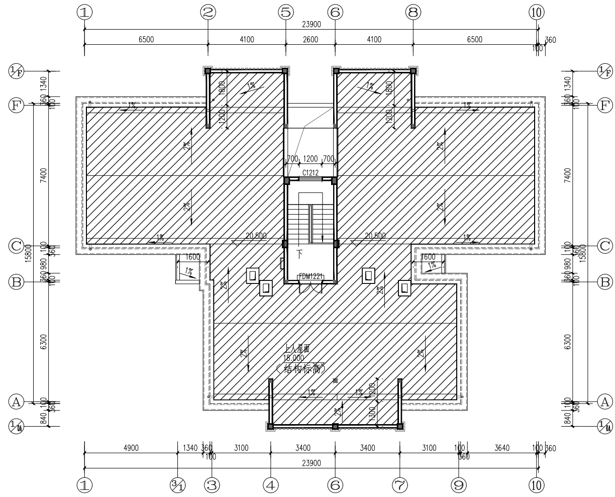
7#、12#屋顶平面改造范围示意图
