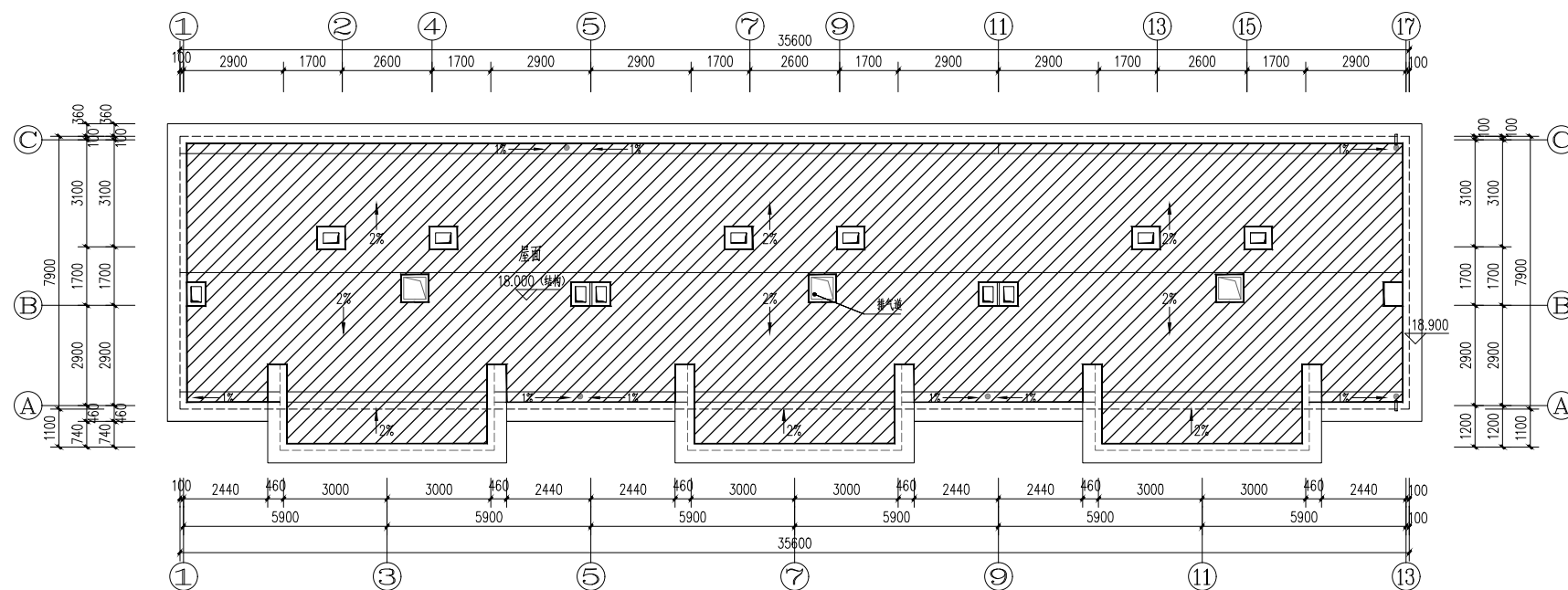
4#屋顶平面改造范围示意图
