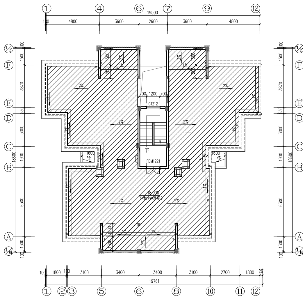
8#、10#、11#标准单元屋顶平面改造范围示意图
