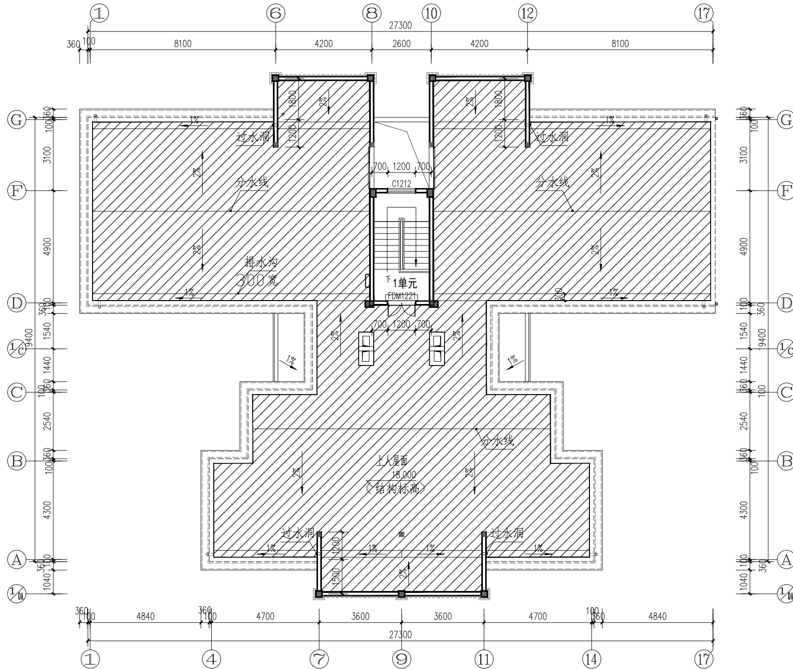
9#、16#标准单元屋顶平面改造范围示意图
