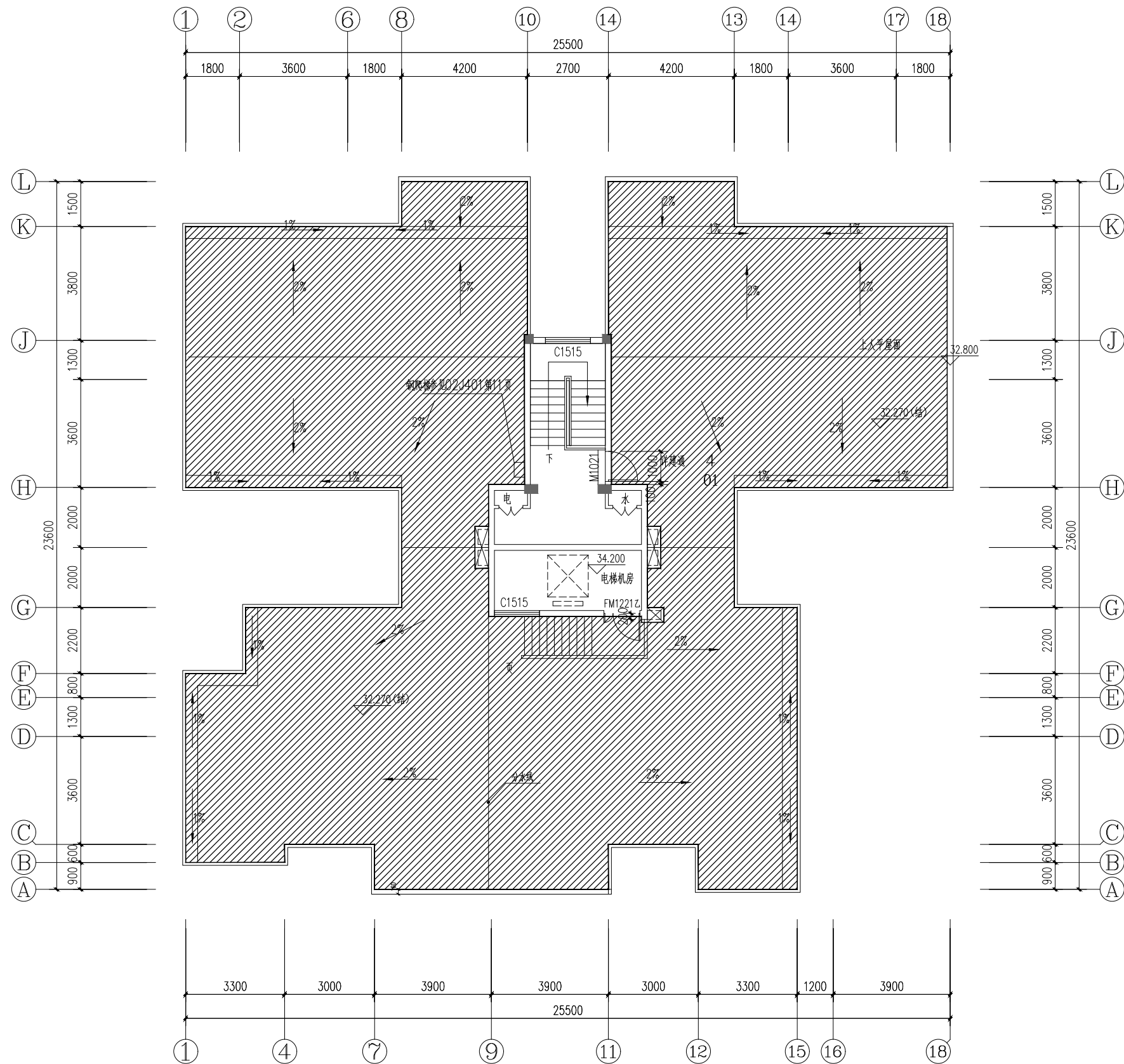
1#、2#、8#标准单元屋顶平面改造范围示意图
