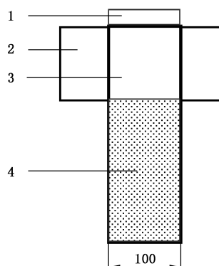
图 H.3 剥离强度试样现场裁取尺寸示意图
