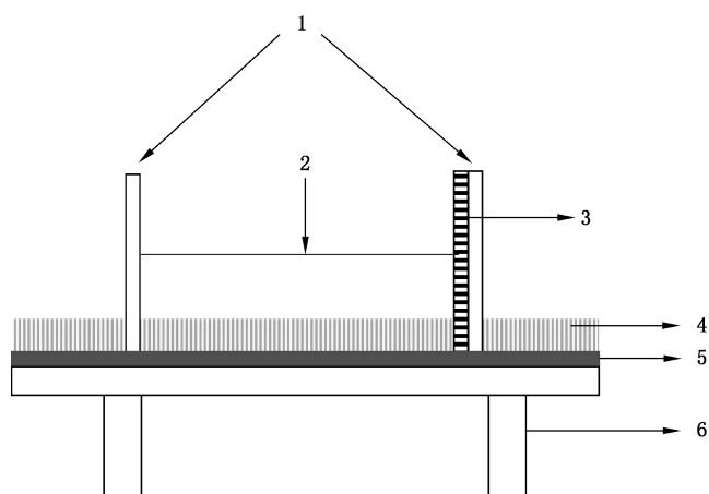
图 G.2 填充式人造草面层渗水速率测试示意图
