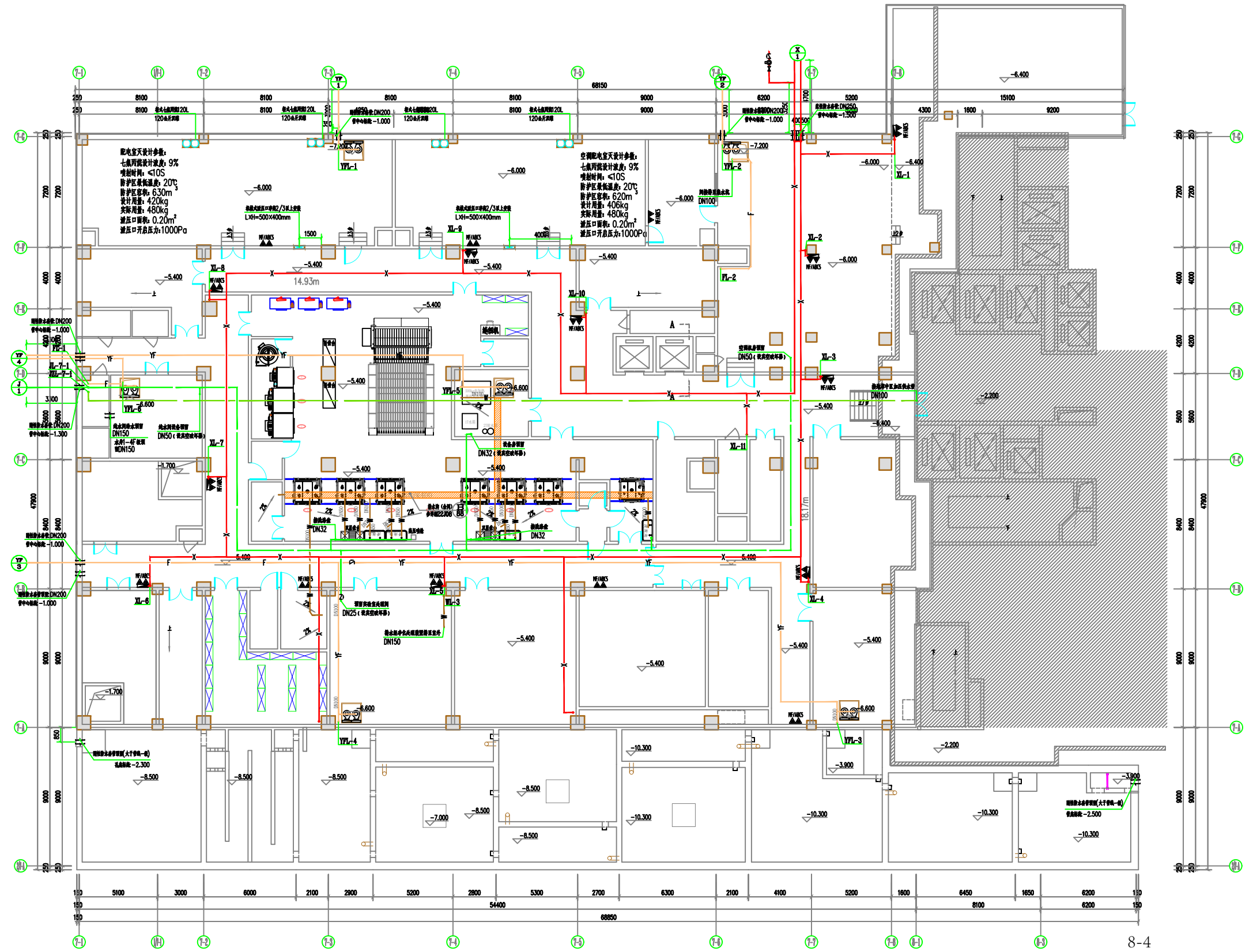
地下一层给排水平面图 1:100
