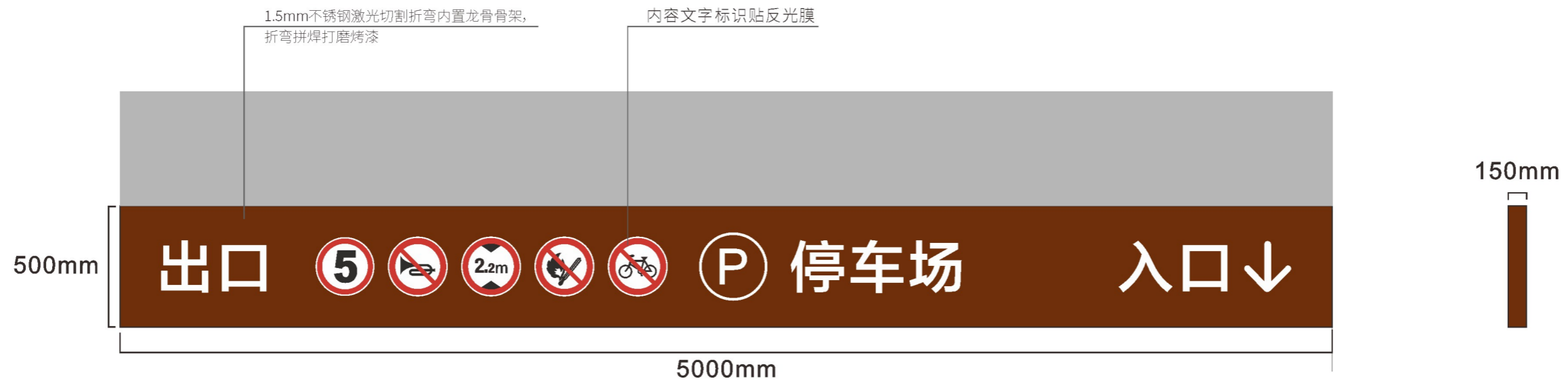
■ 正视图
