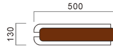
■ 俯视图
